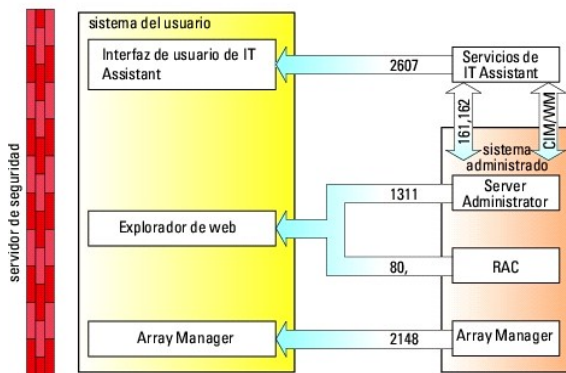
Ilustración 11-1. Instalación típica detrás de un servidor de seguridad
